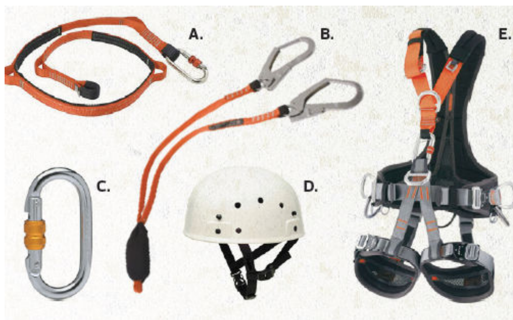
Figura 07: equipamentos para trabalho em altura. FONTE: Manual técnico de poda de árvores, Prefeitura de São Paulo, 2012.
