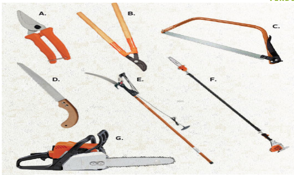
Figura 04: Ferramentas de poda. FONTE: Manual técnico de poda de árvores, Prefeitura de São Paulo, 2012.
