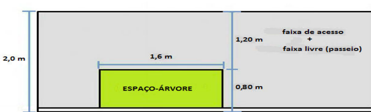
Figura 03: desenho representativo de como se deve realizar o "espaço árvore" em uma calçada de 2 metros.
